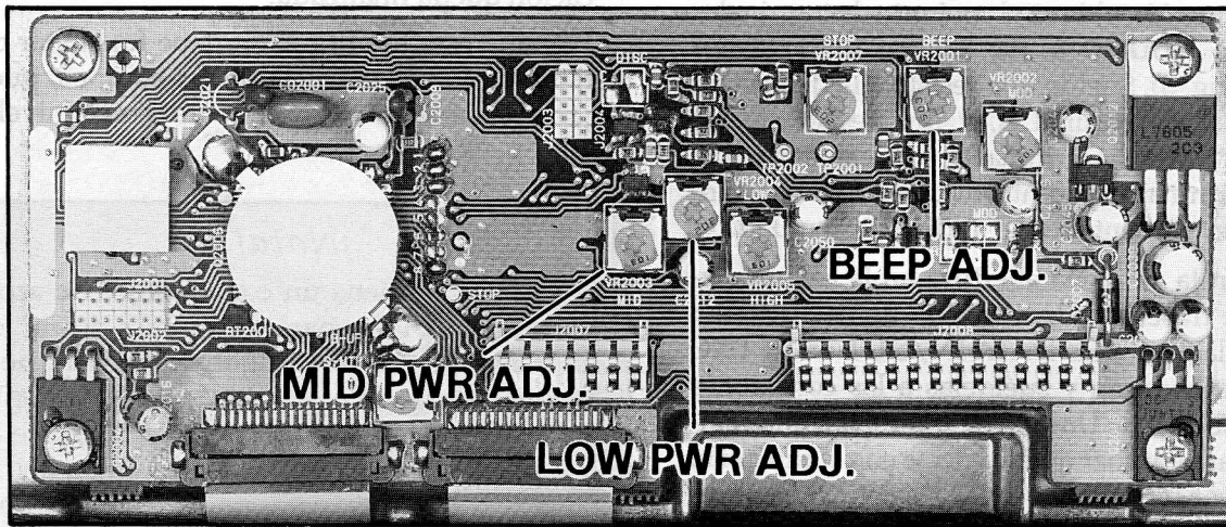
FT-2500M Localización de Ajustes Internos
