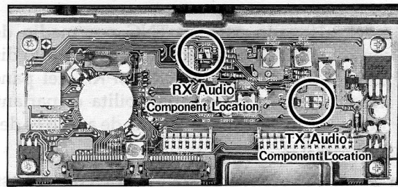
Fig. 1 Ubicación de Componentes para Modificaciones
